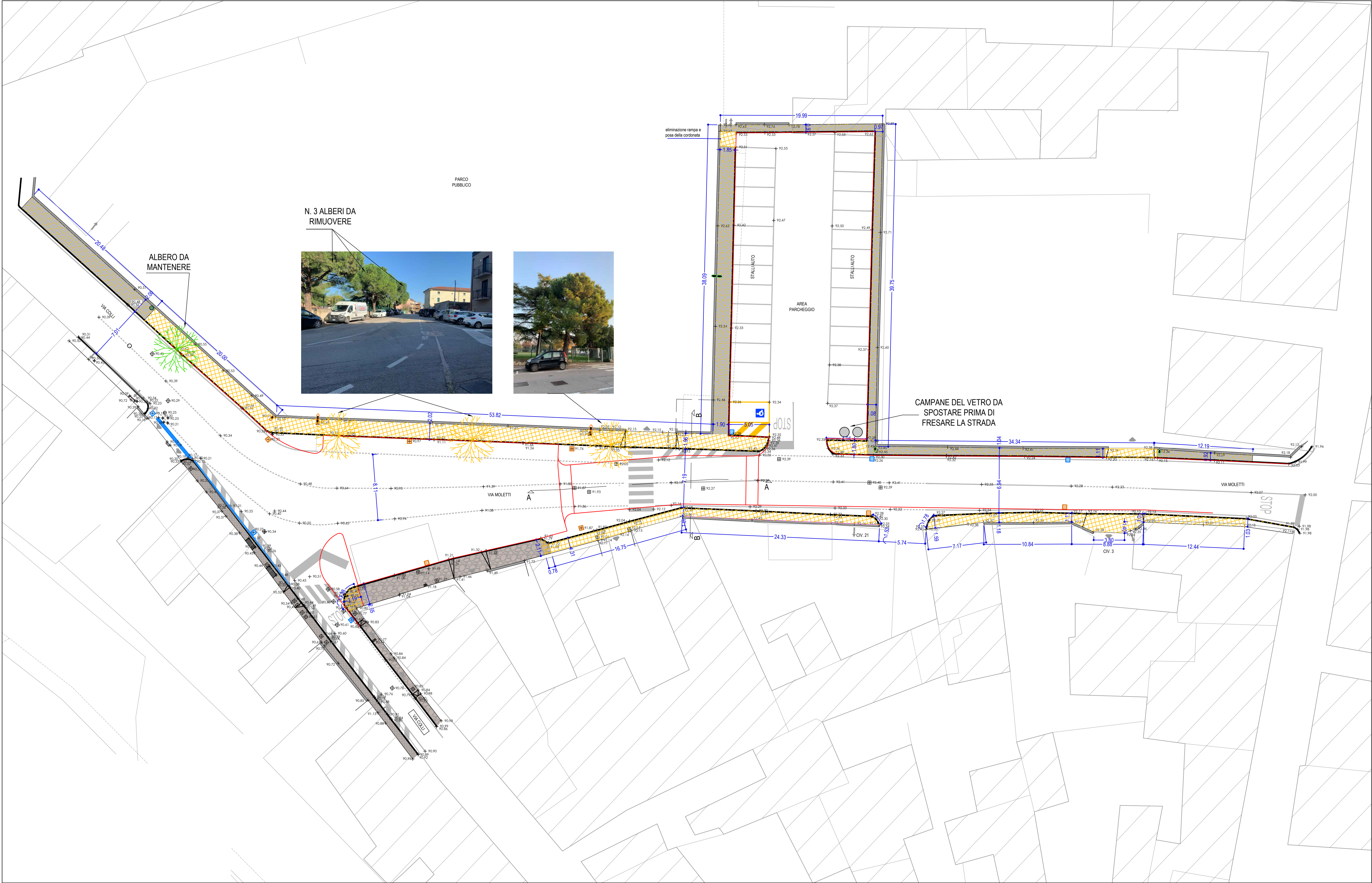
PLANIMETRIA STATO ATTUALE E RILIEVO PLANO-ALTIMETRICO scala 1:250
